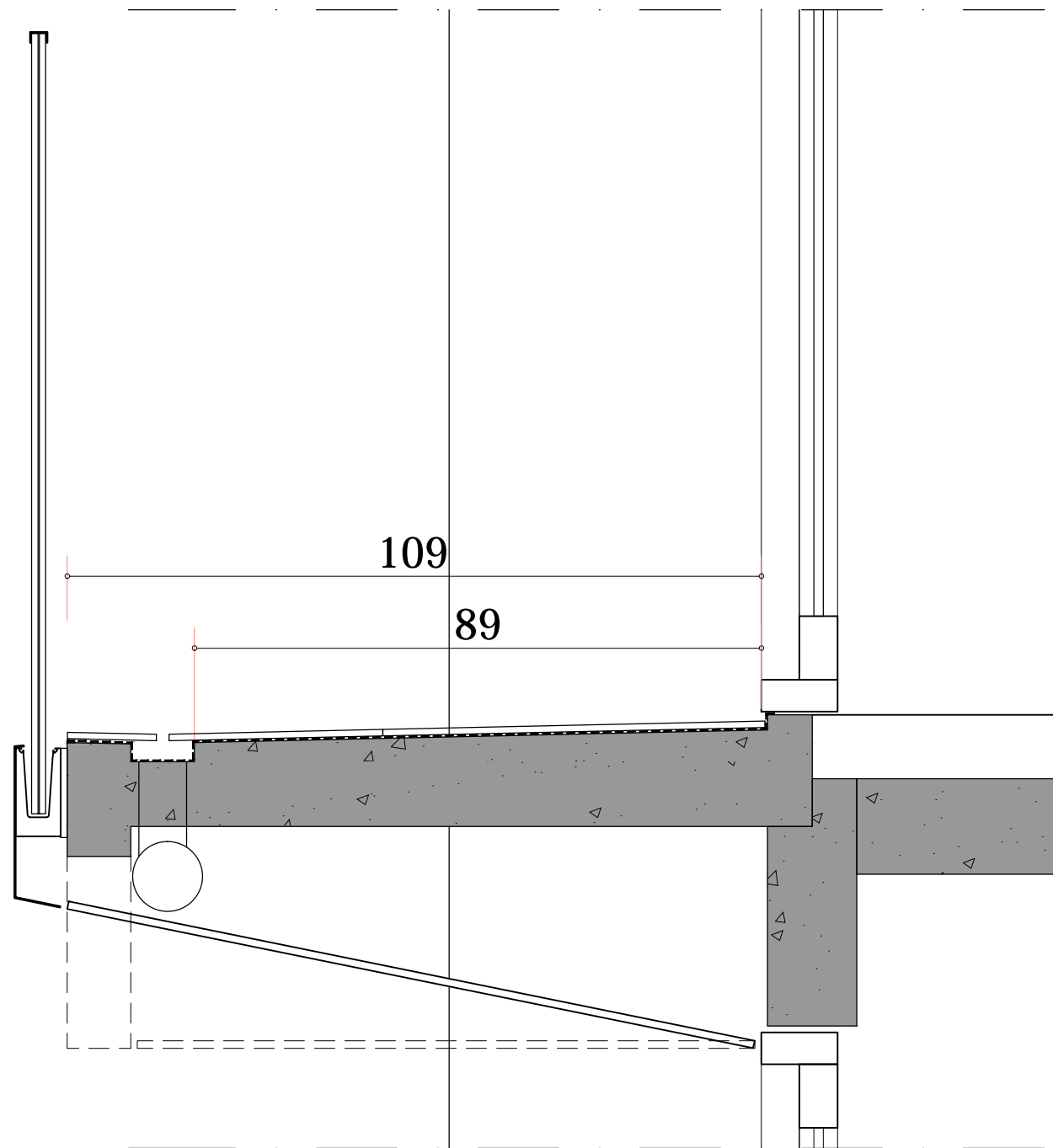
Nieuwe toestand optie 1
