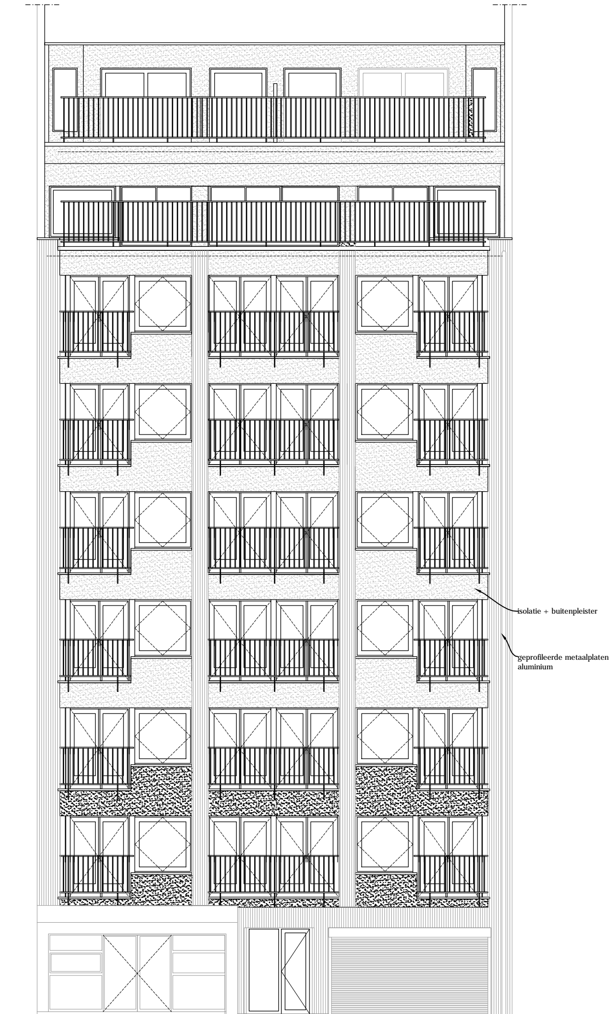
BESTAANDE TOESTAND Voorgevel
